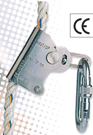
ANTI-CHUTE MOBILE STOP LIGHT GUIDED FALL ARRESTER STOP LIGHT DISPOSITIVO ANTICAIDAS MOVIL CON CUERDA
